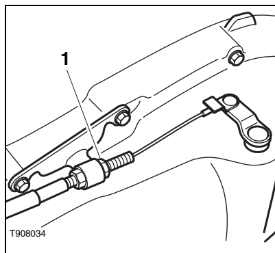
1. Dispositif de réglage (extrémité moteur)
